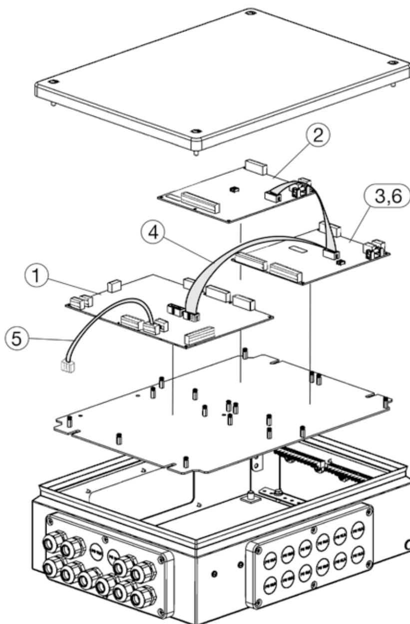
Afbeelding 22: Reserveonderdelen schakelkast
