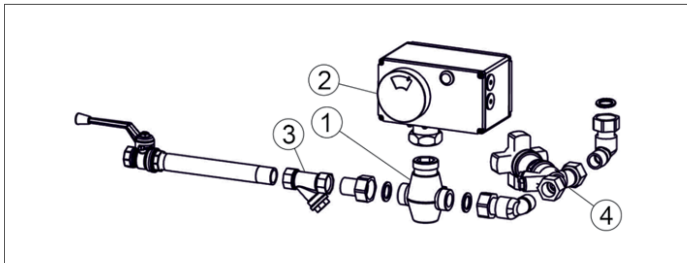
Afbeelding 24: Ontgassingsmodule EMAE
