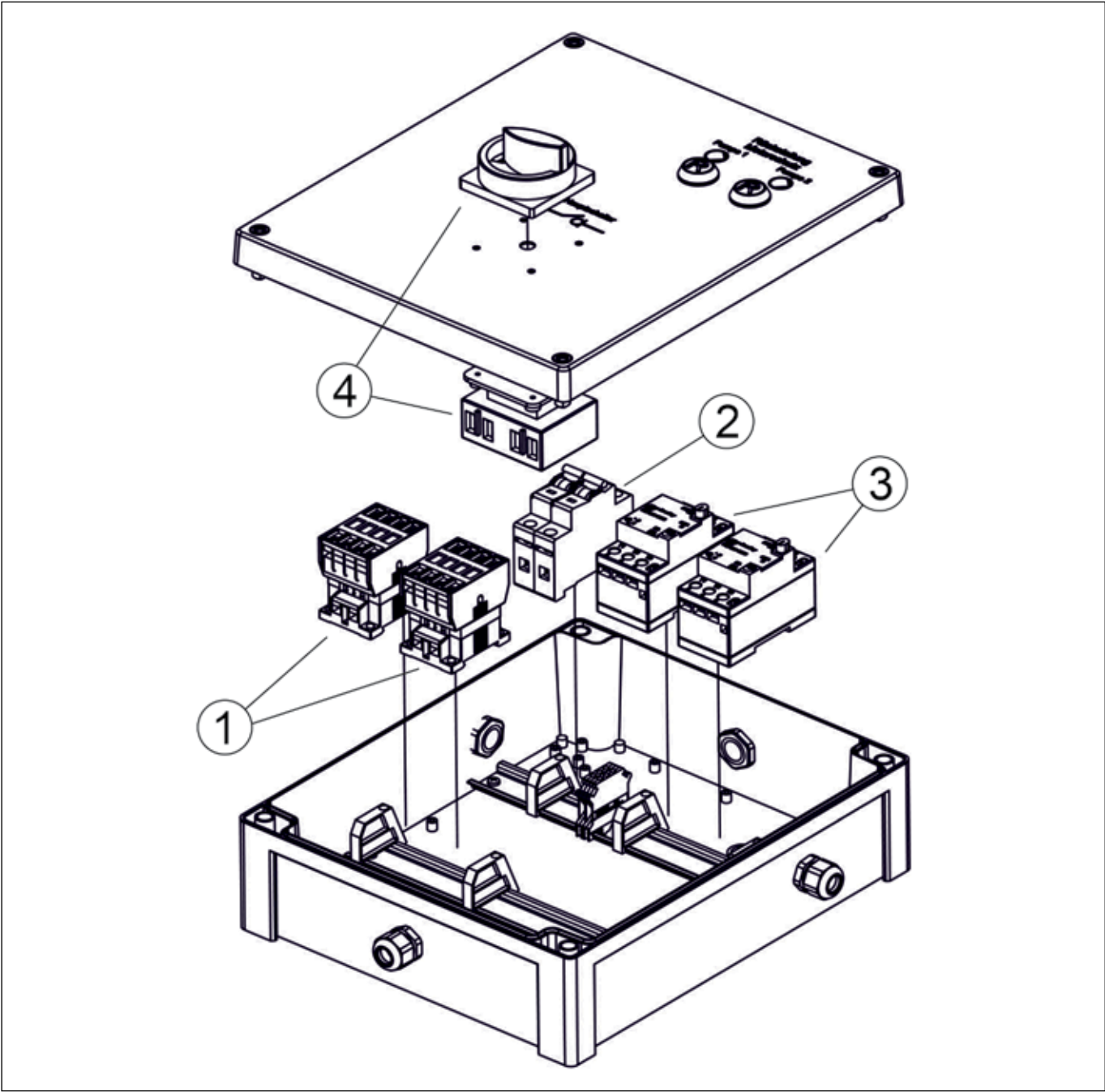
Afbelding 25: Vermogensdeel
